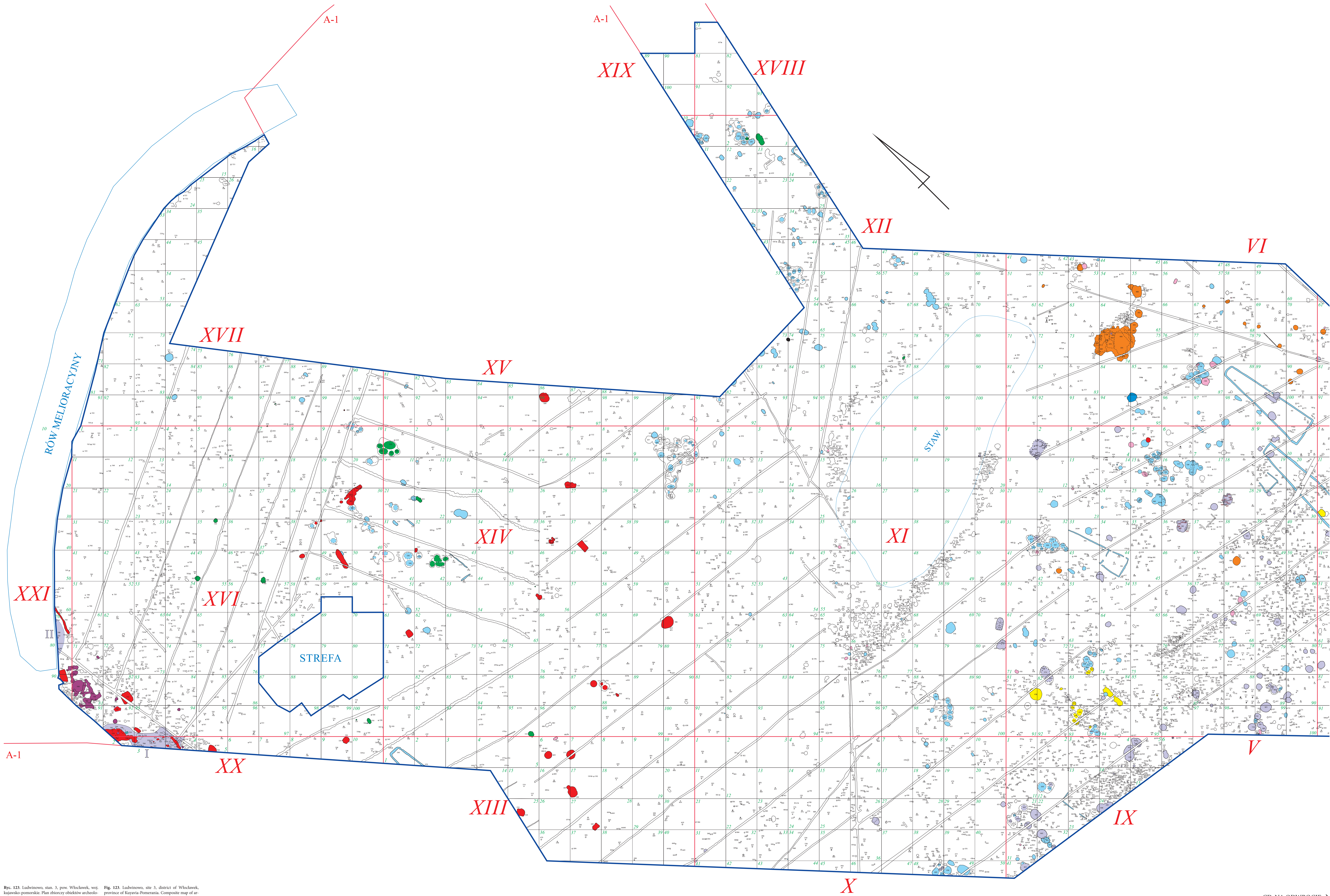
Ryc. 123. Ludwinowo, stan. 3, pow. Włocławek, woj. kujawsko-pomorskie. Plan zbiorczy obiektów archeologicznych z podziałem chronologicznym.
